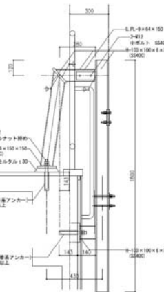
壁面固定式バスケットゴール受材詳細図と 補強後のバスケットゴール
